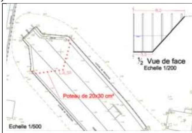
Figure 7 : Dispositif anti-embâcles proposé sur un canal de délestage des eaux de crue en milieu urbain.
